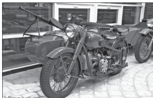
Мотоцикл М-20
